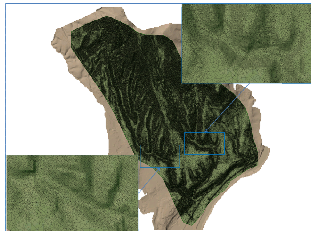
Exemple de maillage de calcul bidimensionnel adapté aux variations de la topographie
